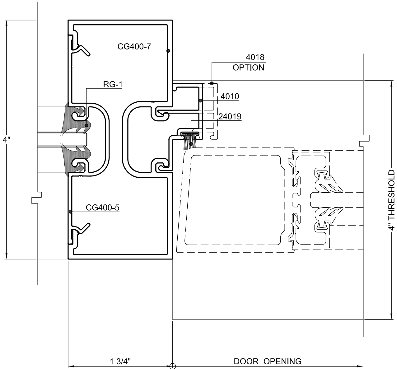
40 DOOR JAMB
